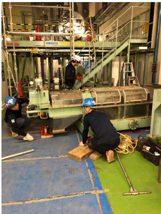
既設前処理設備撤去①(R2. 6. 6)
