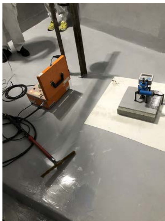
防食塗膜工事完成検査①(R2. 9. 25)
