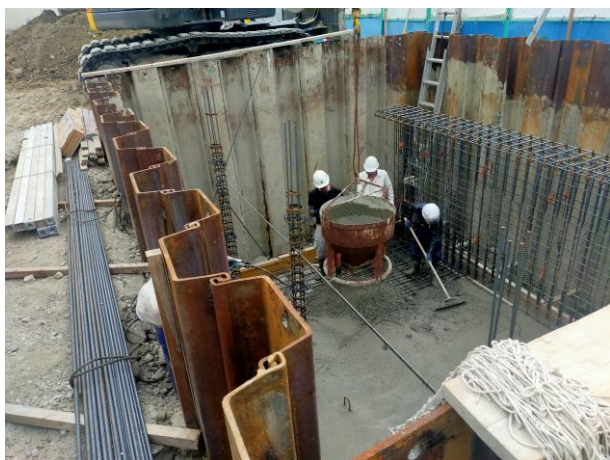
▶コンクリート打設工事②(R8. 8. 17)
